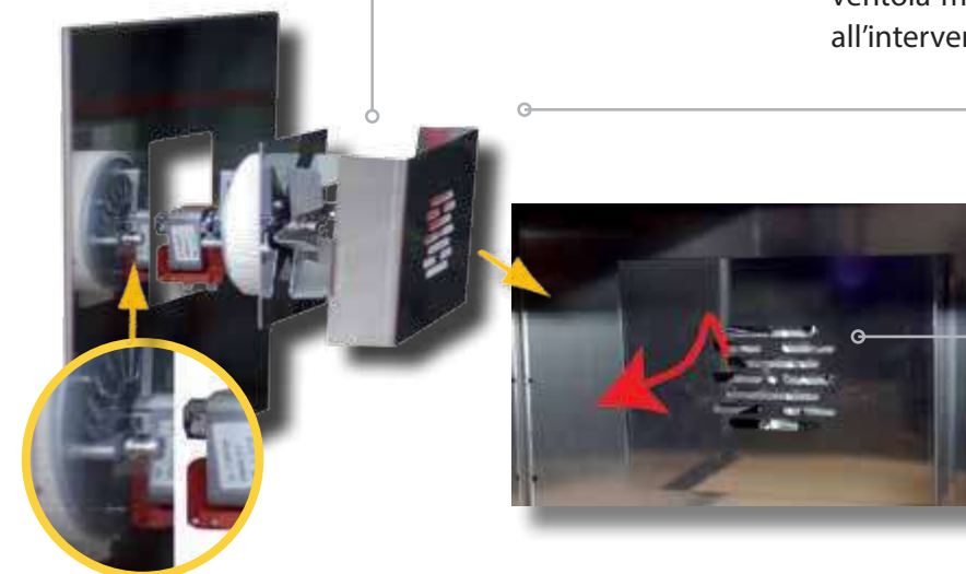
Il fondo della camera di cottura con la flangia da sganciare.
